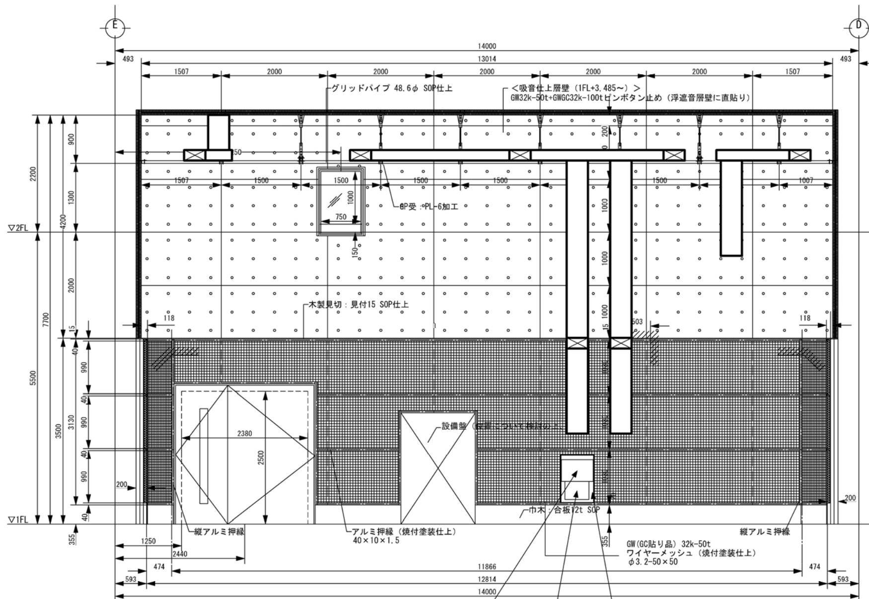
B 展開図 S=1/30
